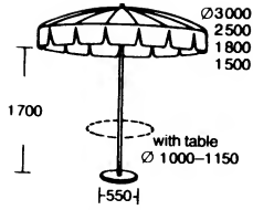
2 Sunshade
